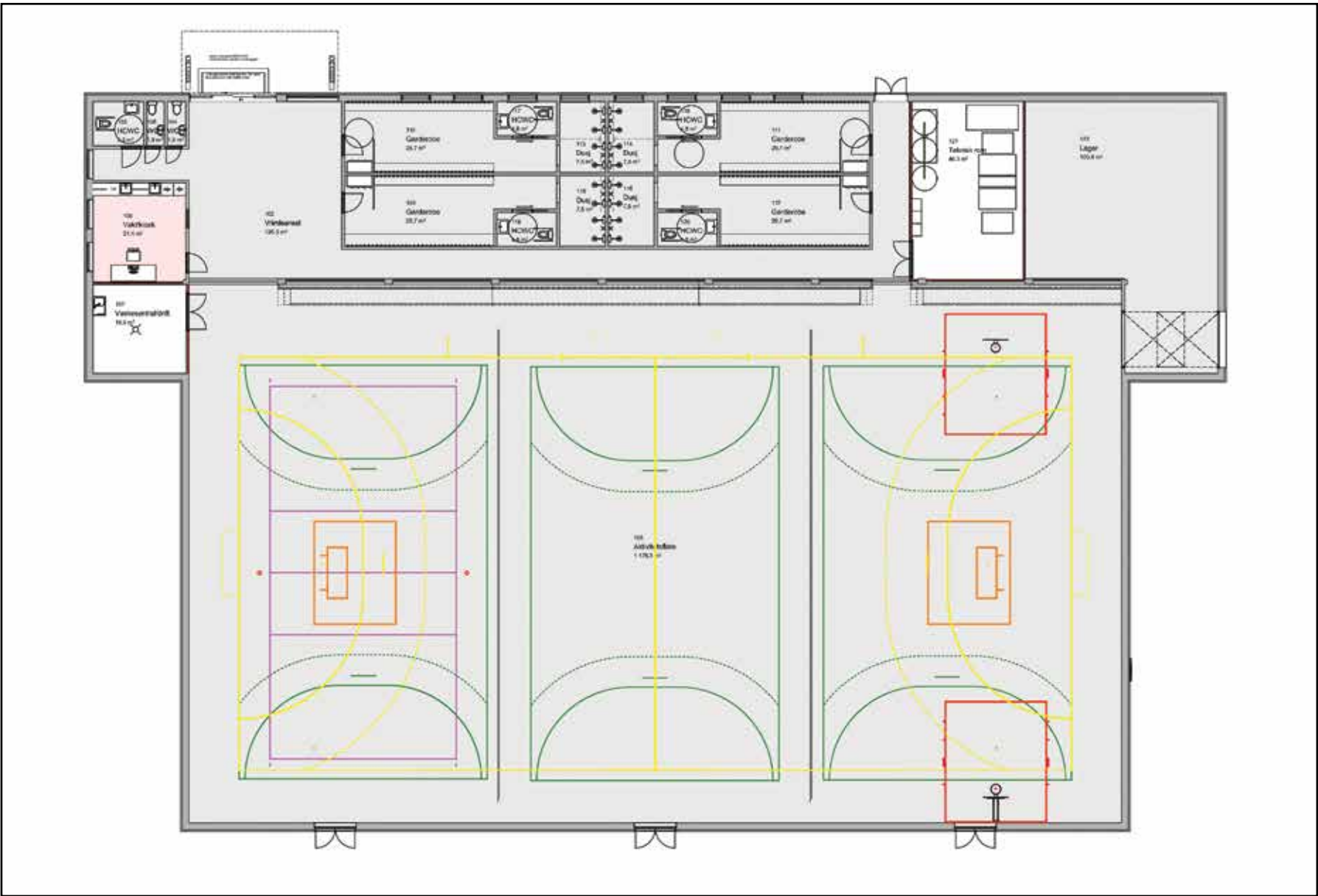
PLANTEGNING - INNE I HALLEN.
