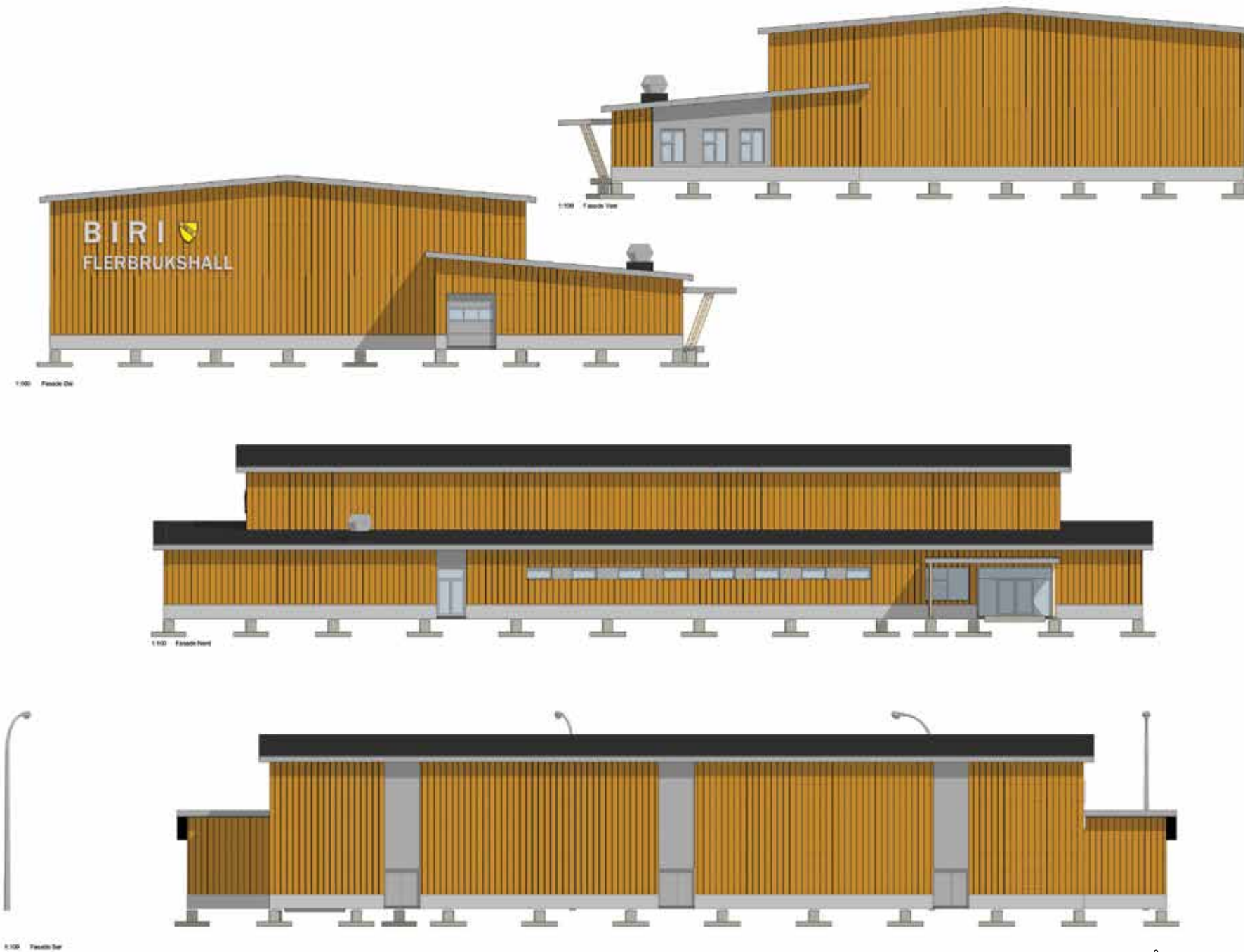
FASADER PÅ HALLEN
